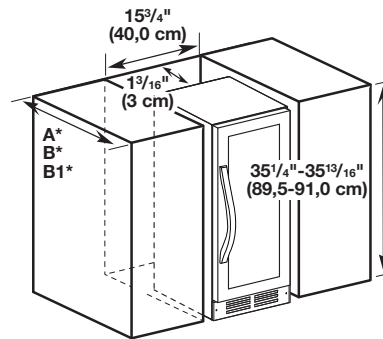
WUW35X15DS WUW55X15DS
