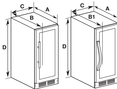
WUW35X15DS WUW55X15DS
